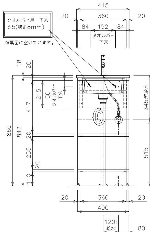
正面図
